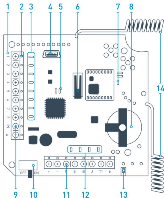
Image 1. Récepteur de capteurs sans fil ocBridge Plus
